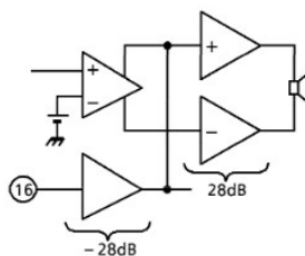
(Fig.6) AUX. amplifier
