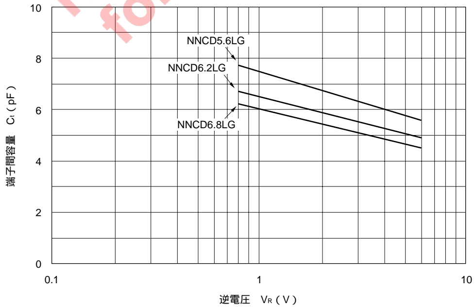
图3 C_t - V_R 特性 ( f = 1 MHz)
