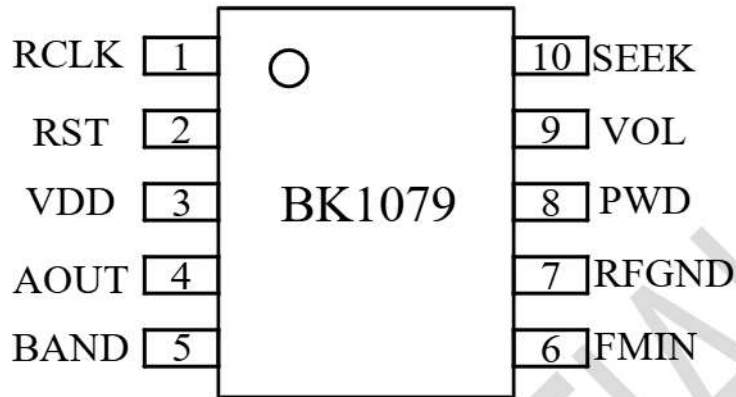
图 1 MSOP10 和 SSOP10 管脚定义俯视图
