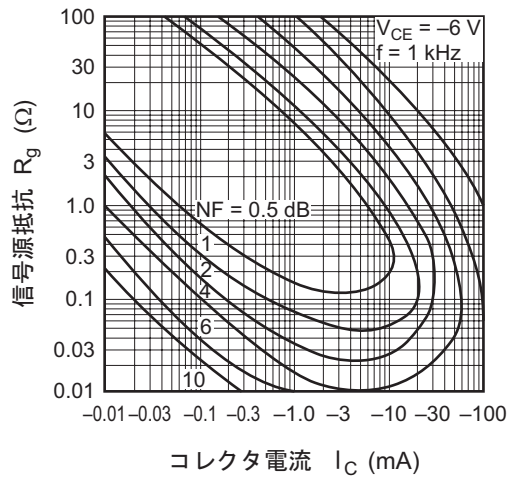
雑音特性 (1)
