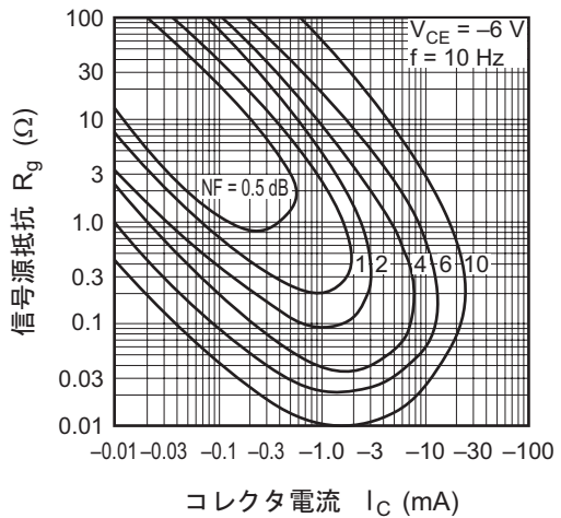
雑音特性 (3)
