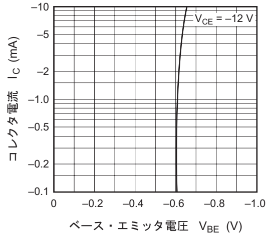
エミッタ接地伝達静特性
