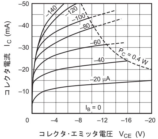
エミッタ接地出力静特性 (1)
