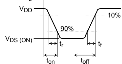
(c) 出力波形 V_{DS}
