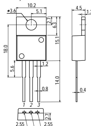
外形図 2010C (unit : mm)
