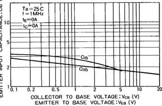
Fig.10 入出力容量—電圧特性
