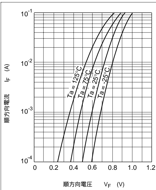
图1. 顺方向特性
