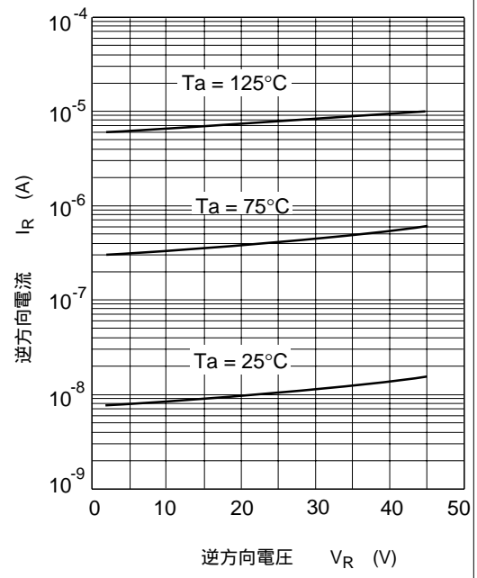
图2. 逆方向特性
